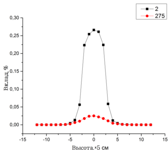
Рис. 9. Вклад в сигнал ДПЗ от 25 зон по высоте ТВС-1 от разных ТВЭЛов (указан номер ТВЭла в ТВС).
