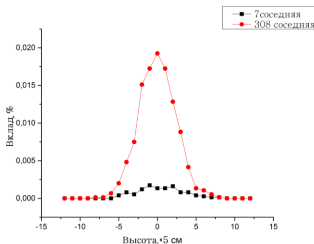
Рис. 10. Вклад в сигнал ДПЗ от 25 зон по высоте ТВС-2 от разных ТВЭЛов (указан номер ТВЭла в ТВС).
