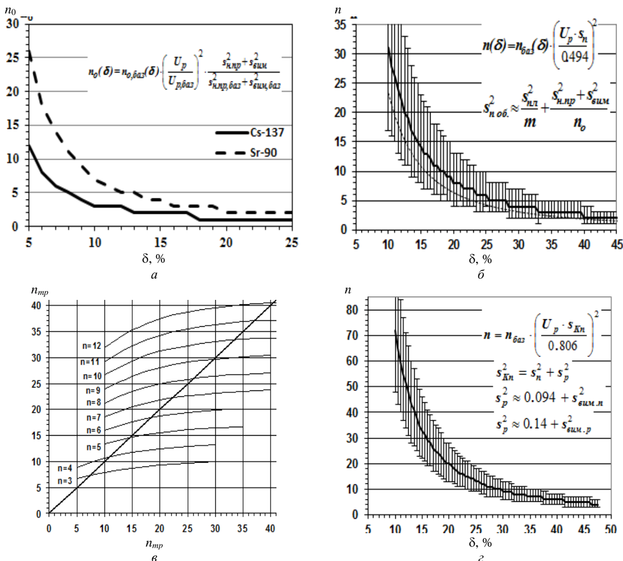
Рис. 3. Мінімально необхідне число відібраних проб і зразків: a - для оцінки медіани активності проби ґрунту з похибкою \delta об'ємом 100 \text{ см}^3 ; б - для оцінки медіани щільності забруднення ґрунту на безградієнтних ділянках; в - для оцінки монотонного тренду щільності забруднення; г - для оцінки медіани коефіцієнта переходу ^{137}\text{Cs}(^{90}\text{Sr}) .
