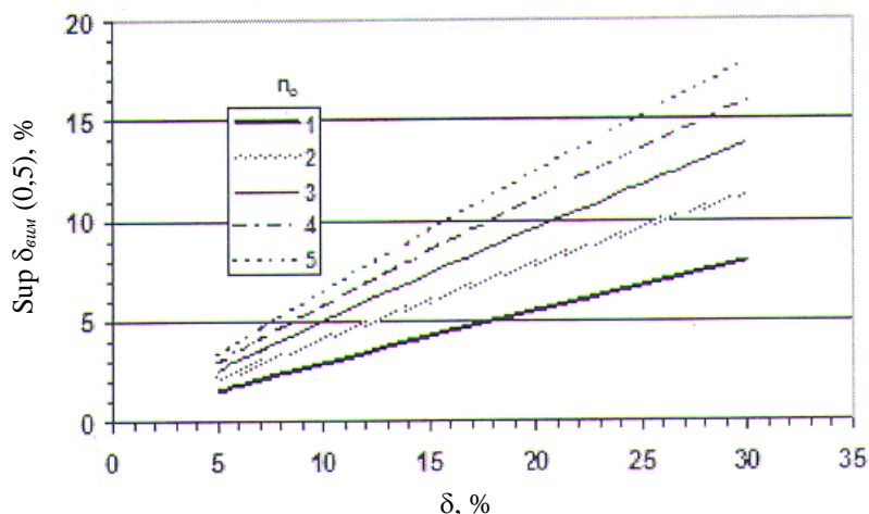
Рис. 4. Граничне значення \delta_{\text{вим}} , що значимо впливає на мінімально необхідне число відібраних проб і вимірювань активності.
