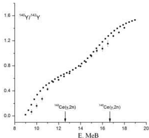
Рис. 3. Експериментальні відношення виходів реакцій (\gamma, n) для ізотопів ^{140}\text{Ce} і ^{142}\text{Ce} .
